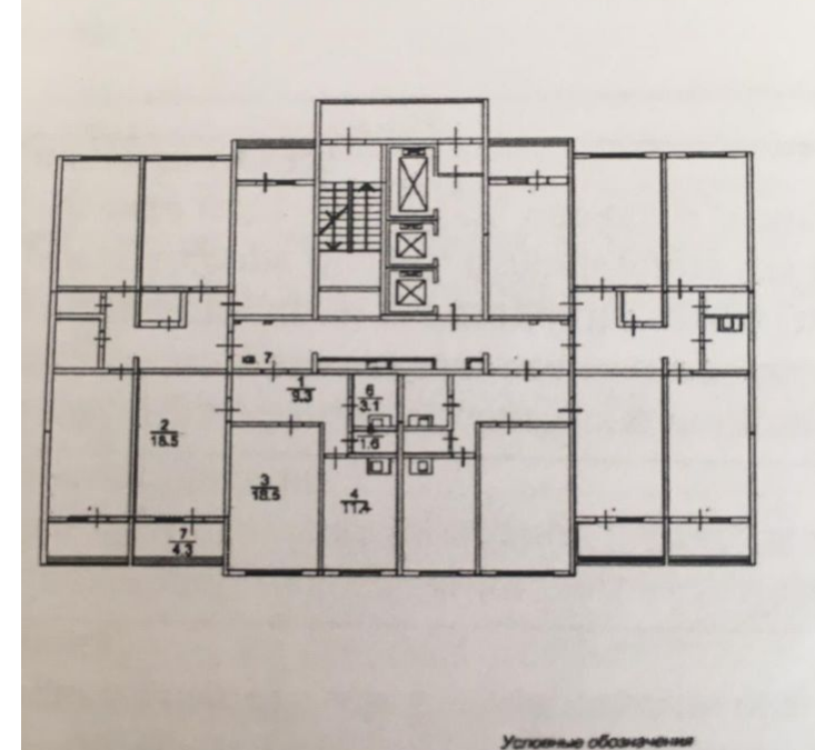
Угловые обозначения
